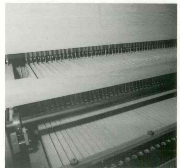
Einarmige Klaviatur mit Trakturausgleich
